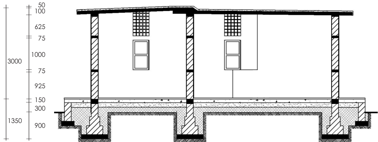
Section D-D
