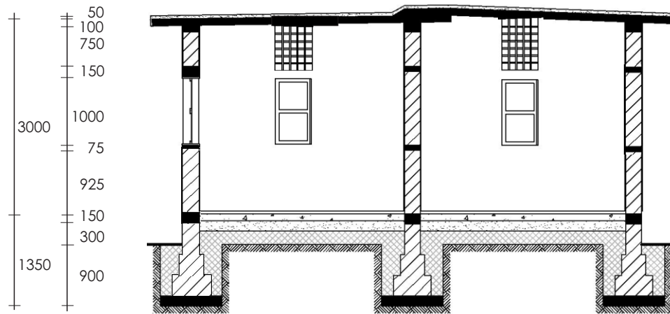
Section D-D
