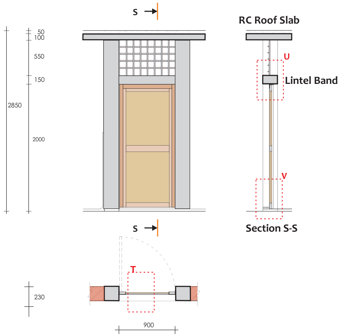
Door Details
