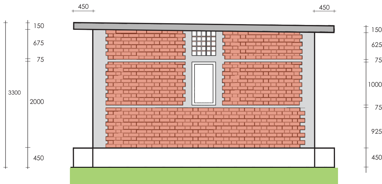
Right Elevation
