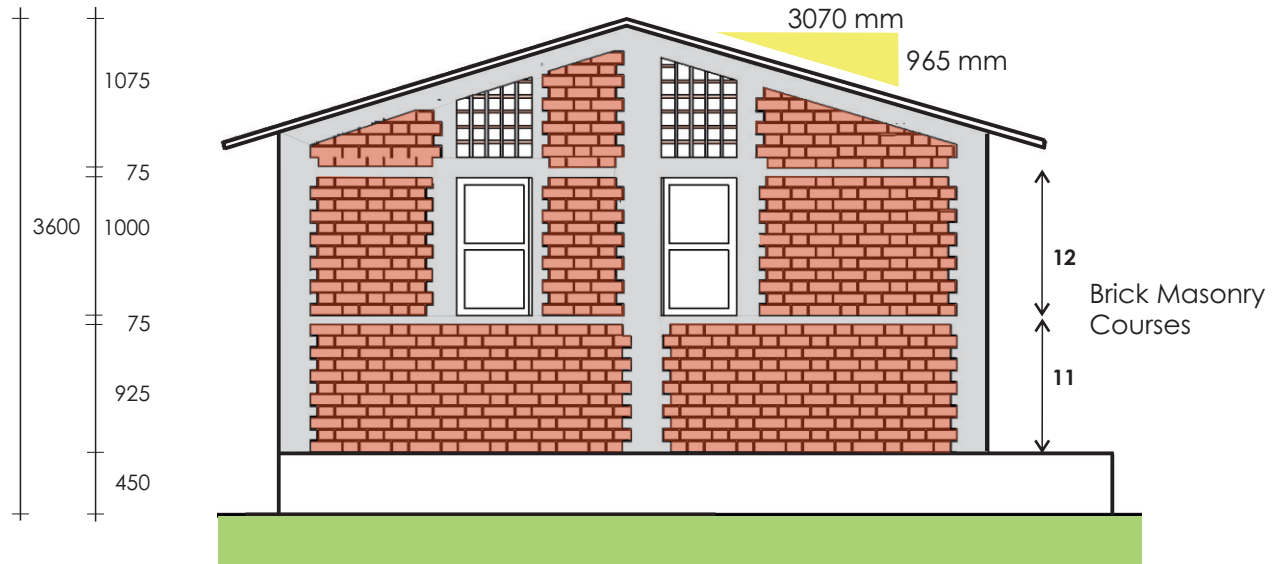
Right Elevation
