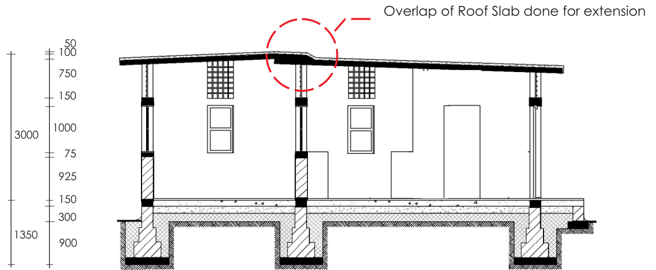
Section D-D
