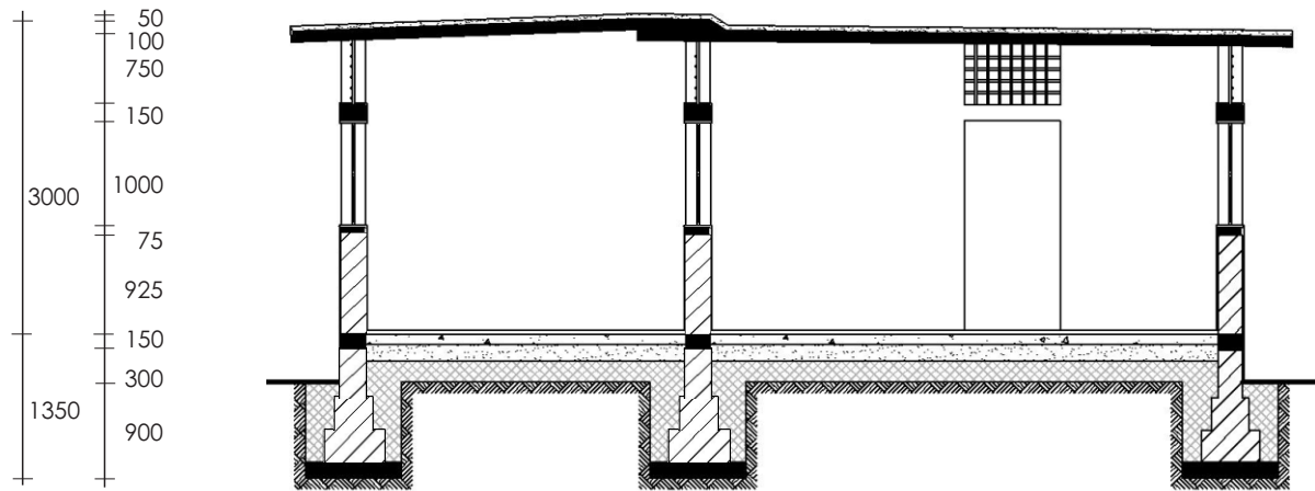
Section D-D
